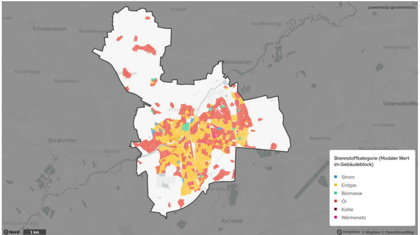
Abbildung 9: Übersicht der eingesetzten Energieträger nach Baublock
