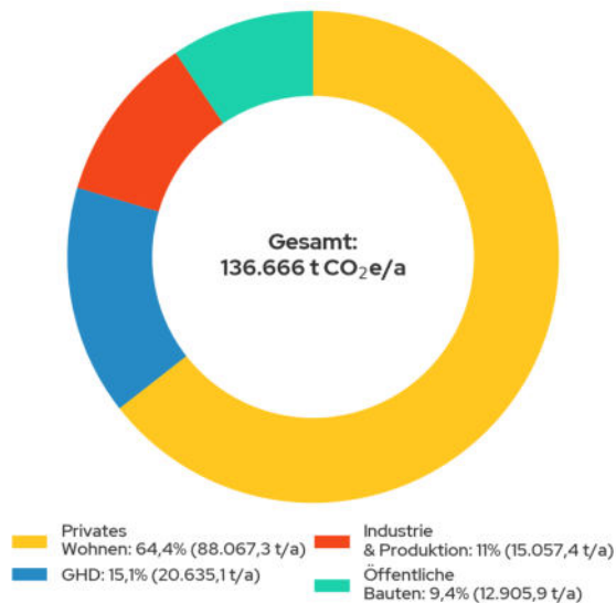
Abbildung 13: Treibhausgasemissionen nach Sektoren im Projektgebiet
