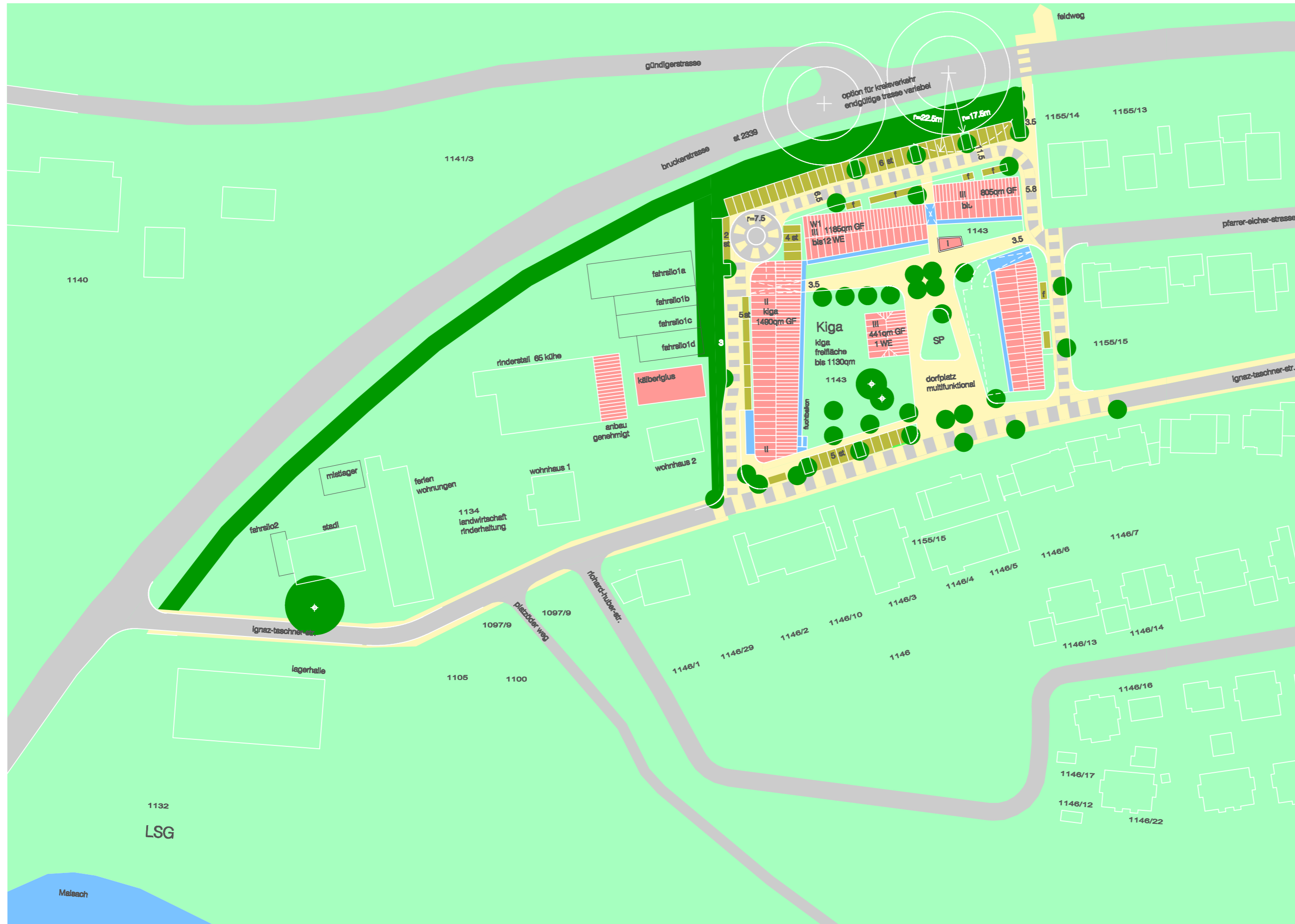
der entwurf ist eine weiterentwicklung des konzeptes der werkgemeinschaft: kath / hendl / schinels var. 2_ek v. 11.04.2017
