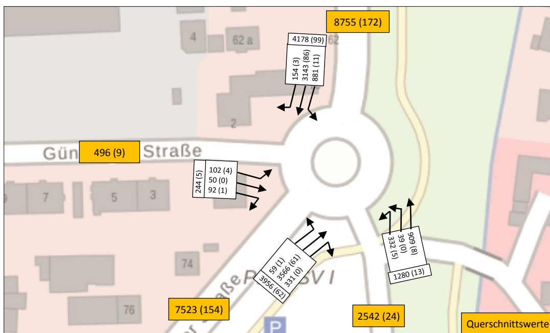
Abbildung 3 DTV-Werte [Kfz (SV)] Prognose-Nullfall 2030 [Kartengrundlage: https://geoportal.bayern.de ]
