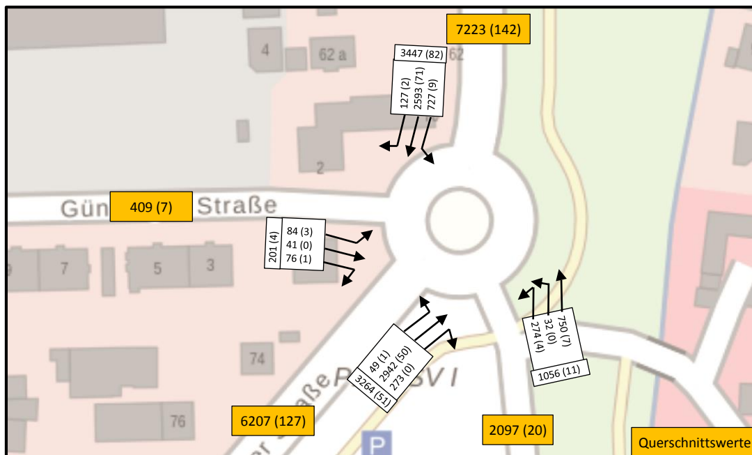
Abbildung 2 DTV-Werte [Kfz (SV)] Verkehrserhebung 04/2019 {Kartengrundlage: https://geoportal.bayern.de }
