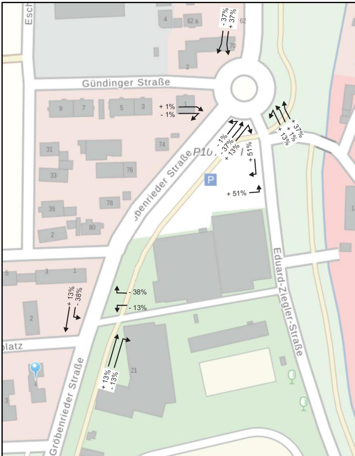
Abbildung 4 Verlagerung des Besucher-/Sportlerverkehrs im Planfall 2030 in [Kfz (SV)] {Kartengrundlage: https://geoportal.bayern.de }
