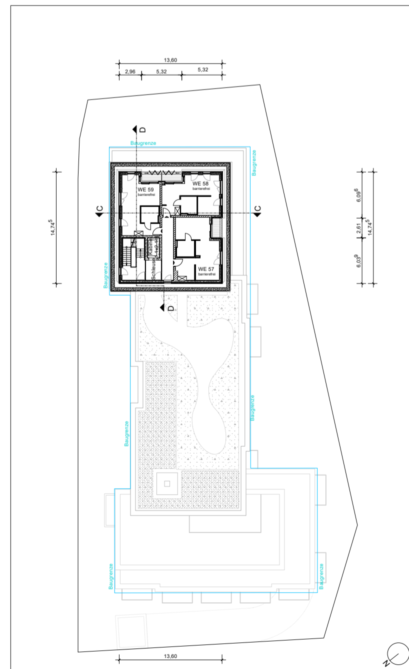
6. Obergeschoss
