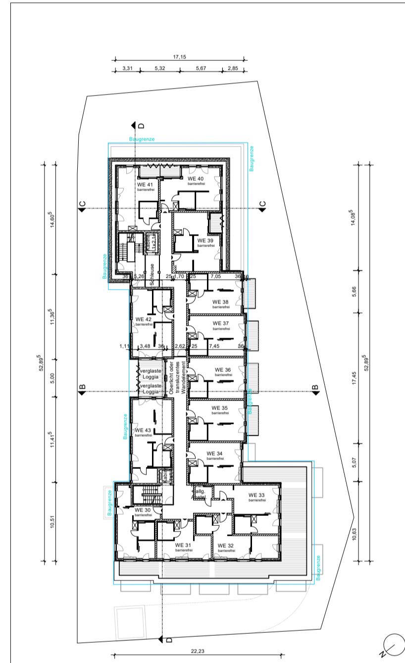
3. Obergeschoss
