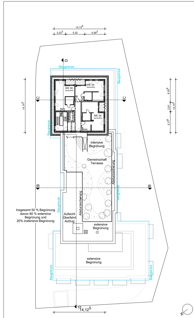
5. Obergeschoss
