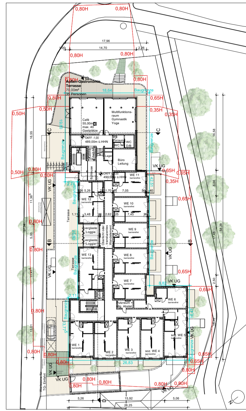
1. Obergeschoss
