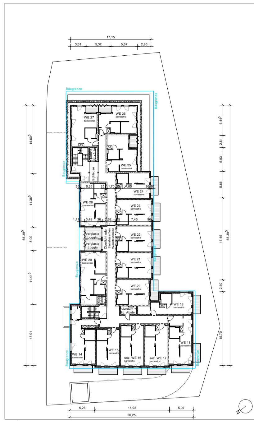
2. Obergeschoss
