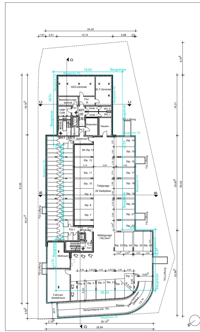
Untergeschoss
