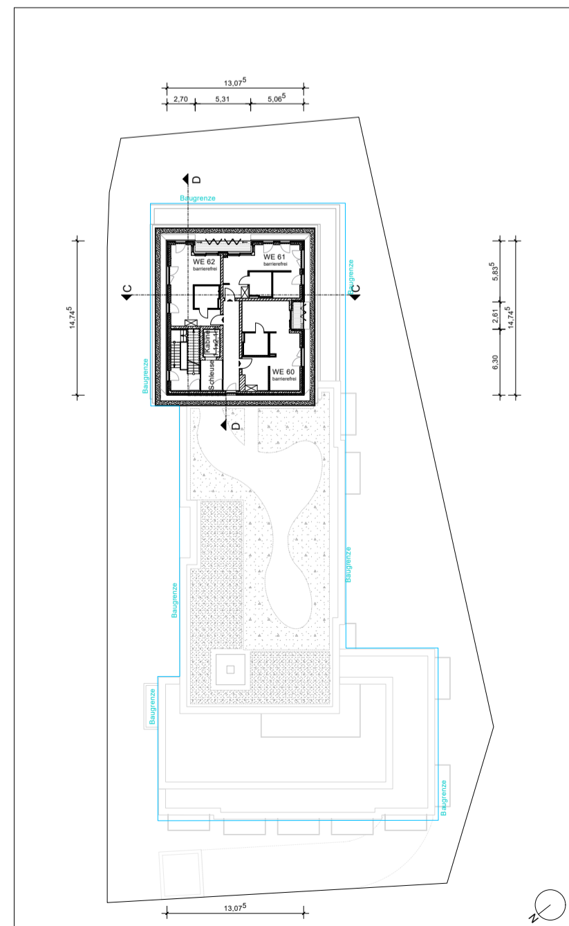
Dachgeschoss
