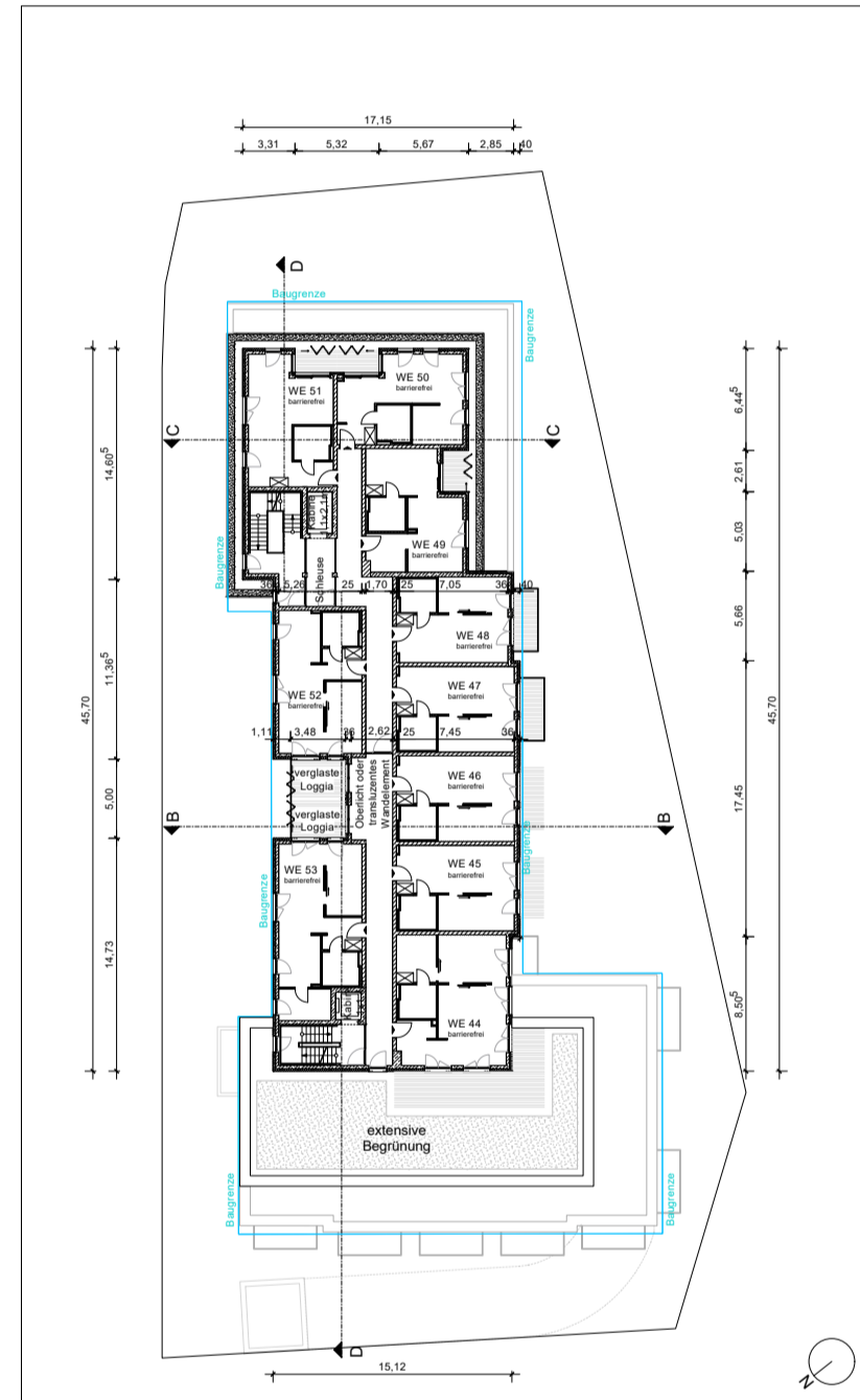
4. Obergeschoss
